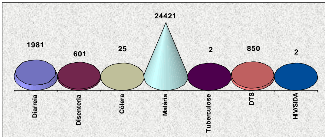
FIGURA 8: Quadro epidémico, 2003
